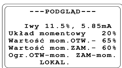
Rys. HH: Podgląd 1
