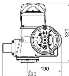
Rys. C: Wymiary siłownika 3XWI
