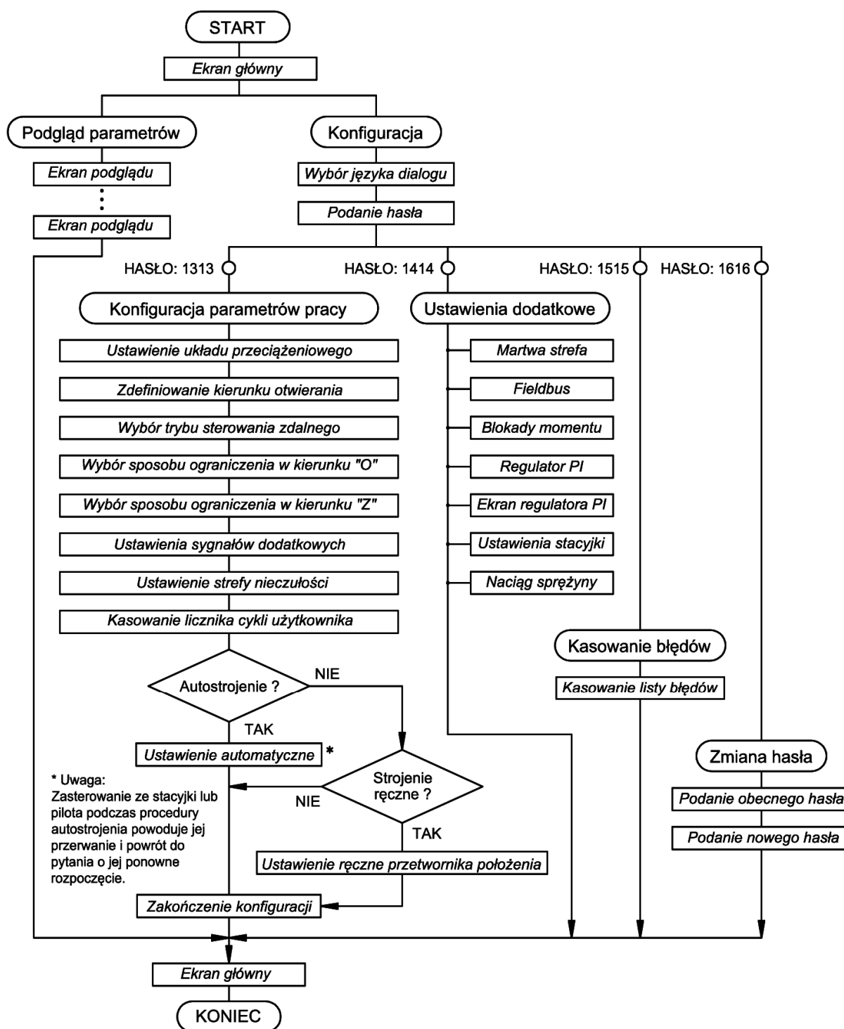
Rys. L: Procedura konfiguracji siłownika
