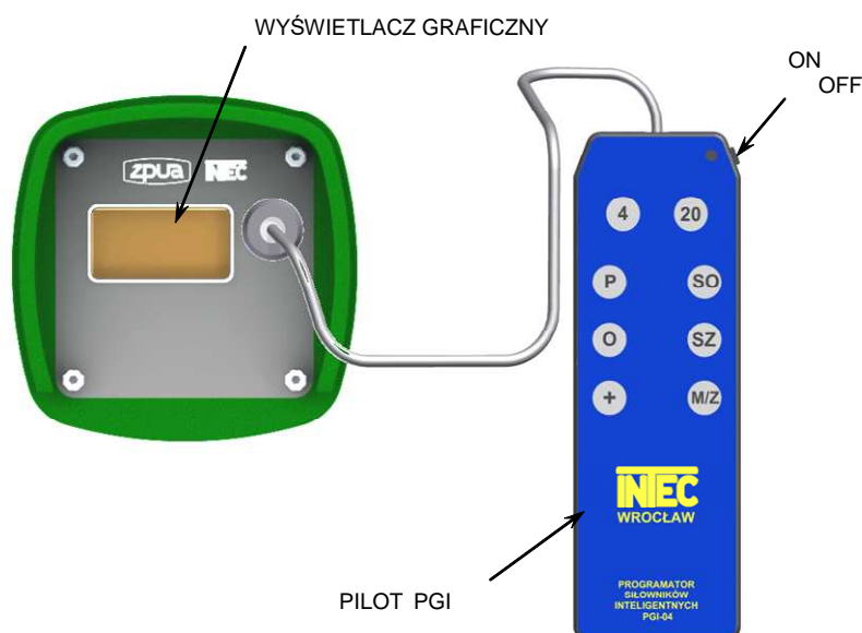
Rys. I: Stacyjka z programatorem
