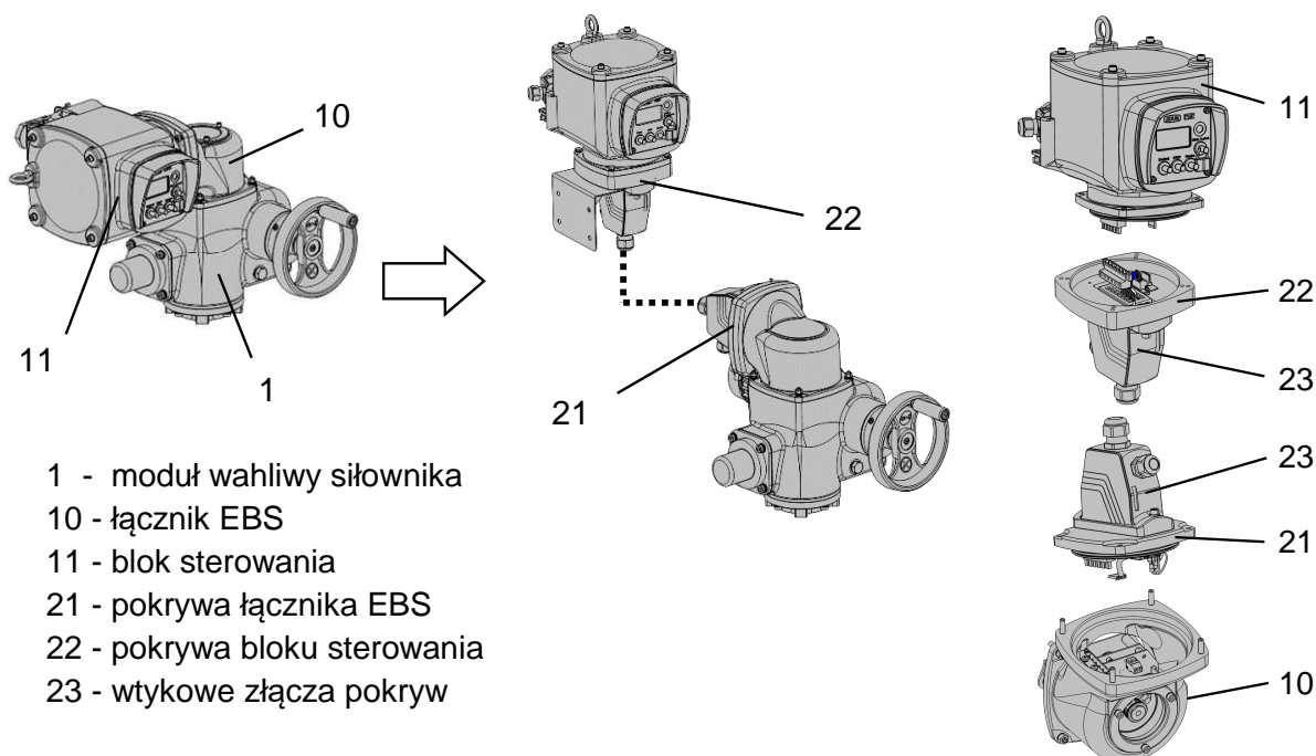
Rys. F: Odsunięcie bloku sterującego
