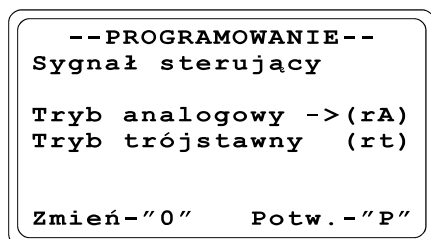
Rys. P: Wybór sterowania
