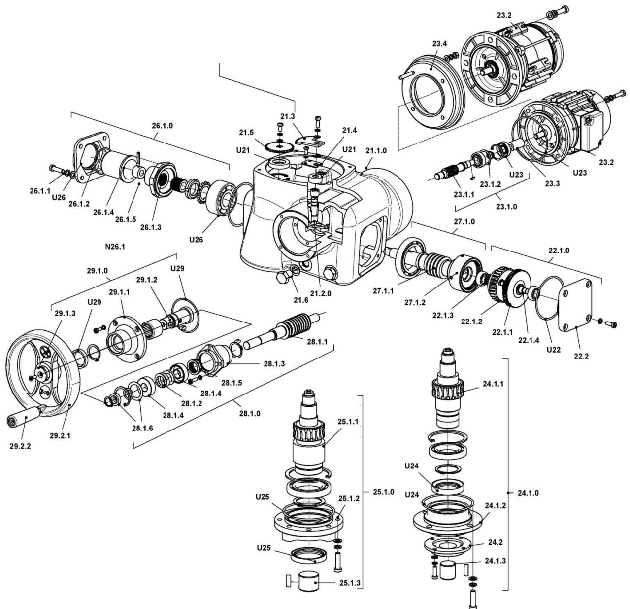
Rys. 00: Części siłownika 3XWI – moduł wahlwy
