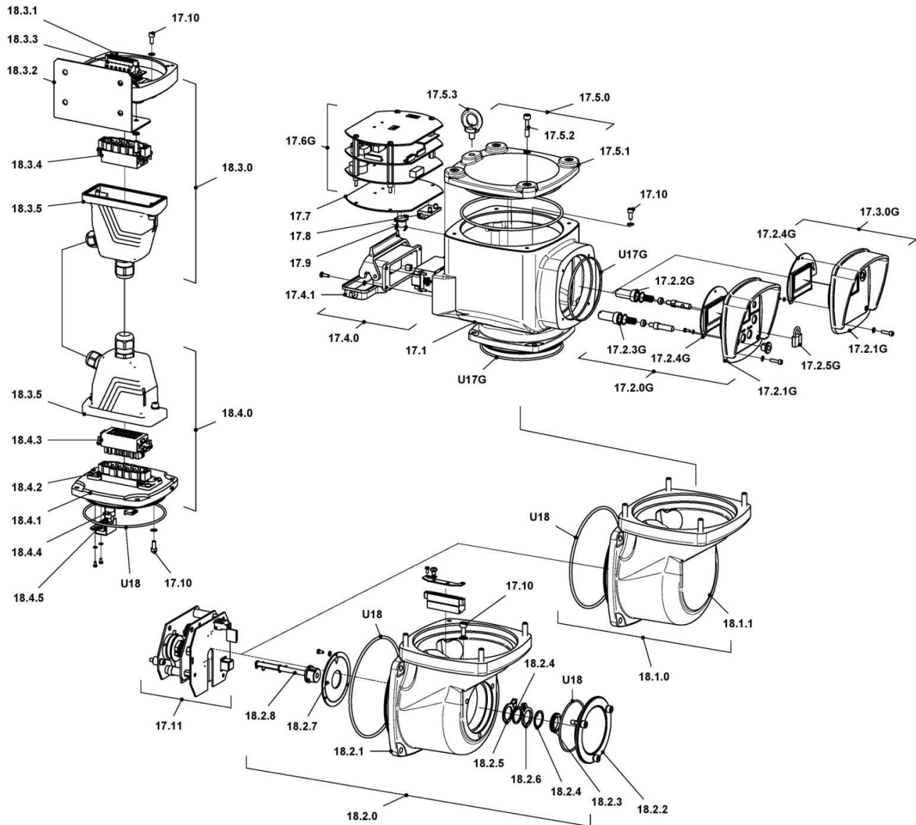
Rys. PP: Części bloku sterowania siłownika 3XWI
