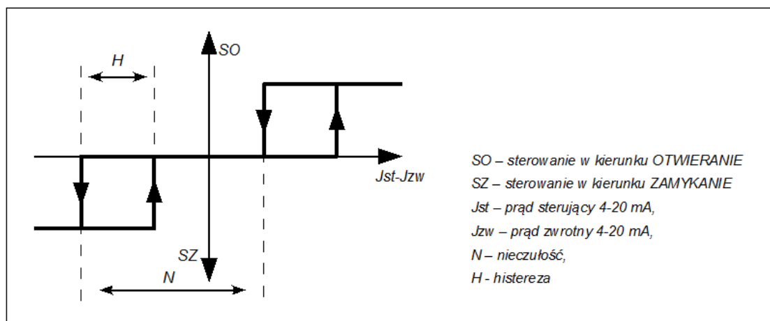
Rys. T: Histereza i strefa nieczułości
