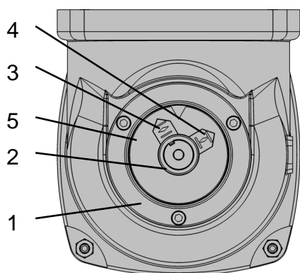
Rys. MM: Mechaniczny wskaźnik położenia
