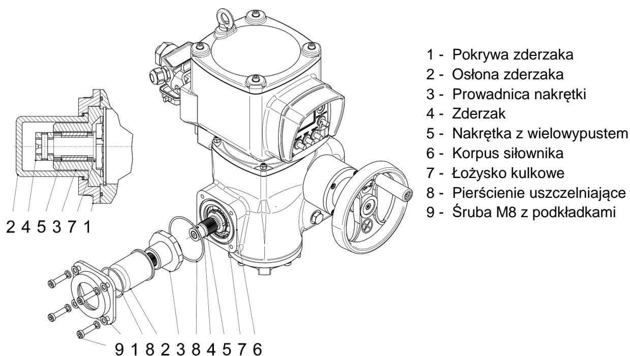
Rys. K: Mechaniczny ogranicznik ruchu
